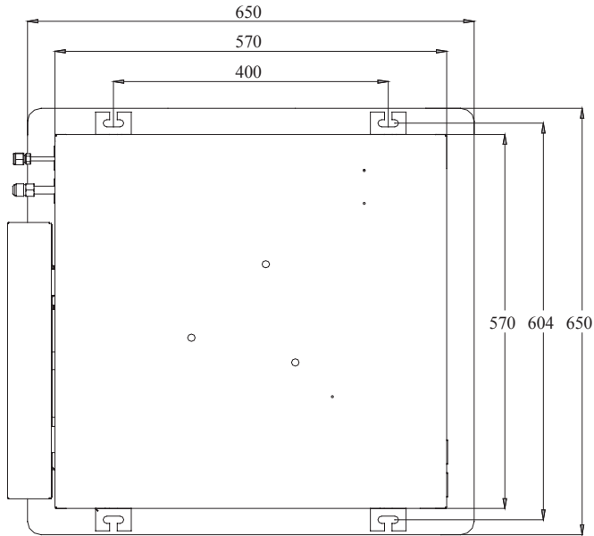
Fig.2 Dimensioni di installazione dei modelli GKH(12)BD-K8DNA5A/T/'GKH(18)BD-K8DNA5A/I
